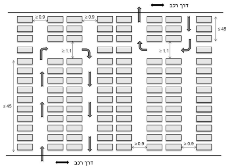
ציור של מערך דרכים בתוך שטח לצורכי קבורה במישור, המאפשר נגישות עד לכל מצבת קבר; המידות במטרים.
